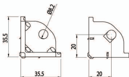
TAPPO TONDO 3 VIE THREE-WAY ROUND CAP TAPÓN REDONDO DE 3 VÍAS BOUCHON ROND 3 VOIES RUNDE DREI-WEGE-ABDECKKAPPE
